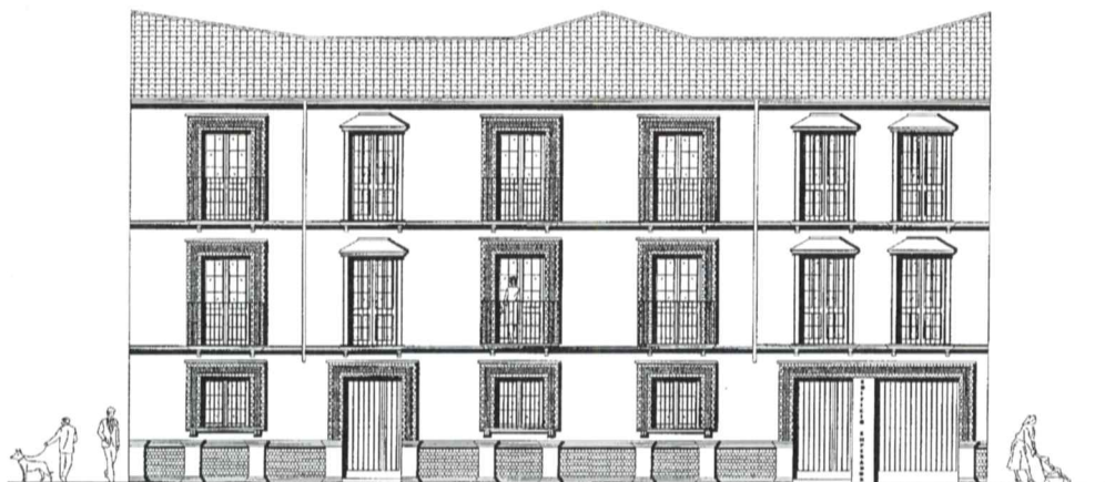
ALZADO CALLE SAN LUIS ARQUITECTO: ANTONIO MARTOS ROJAS
