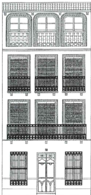
ALZADO CALLE OBISPO CABALLERO. ARQUITECTO: ANTONIO MARTOS ROJAS
